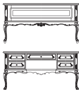
Masa birou Writing desk Письменный стол mm. 1520 x 650 x H.785
