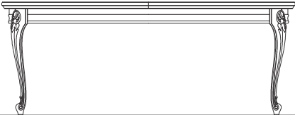
Masa extensibila Extensible table Раздвижной стол mm. 2100/3000 x 1070 x H.770
