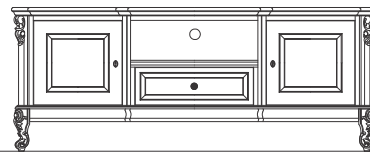
Bufet tv plasma Plasma TV chest Буфет ТВ плазма mm. 1720 x 520 x H.680
