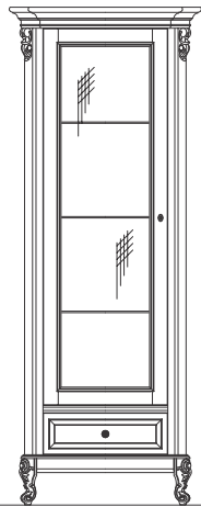
Cristalier 1 usa stanga 1 Door glass cabinet - left Витрина 1 дверь - левая mm. 830 x 590 x H.2140
