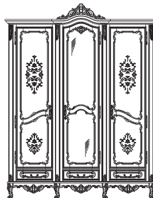
Dulap 3 usi 3 Doors wardrobe Шкаф 3 двери mm. 1810 x 655 x H.2390
