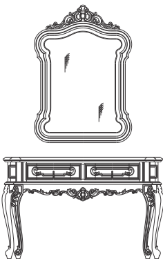
Masa consola Console table Консольный стол mm. 1260 x 420 x H.805
