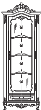
Cristalier 1 usa dreapta 1 Door glass cabinet – right Витрина 1 дверь – правая mm. 800 x 495 x H.2200
